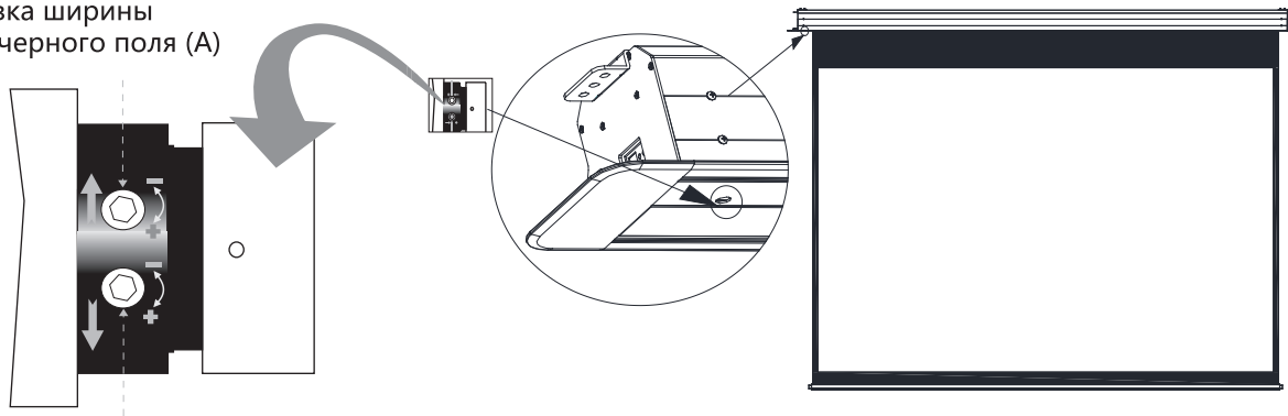
Регулировка положения отвеса при смотке (В)
